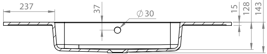
PRZEKRÓJ M-M
